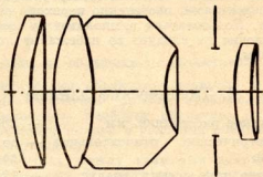
Рис. 1. Оптическая схема объектива.
